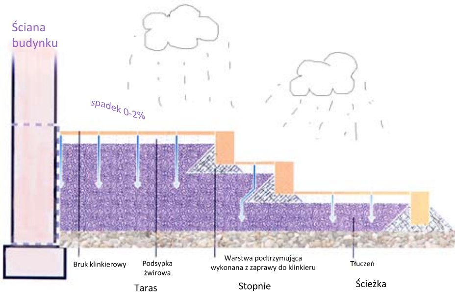
Przekrój tarasu wykonany z bruku klinkierowego na warstwie przepuszczalnej
